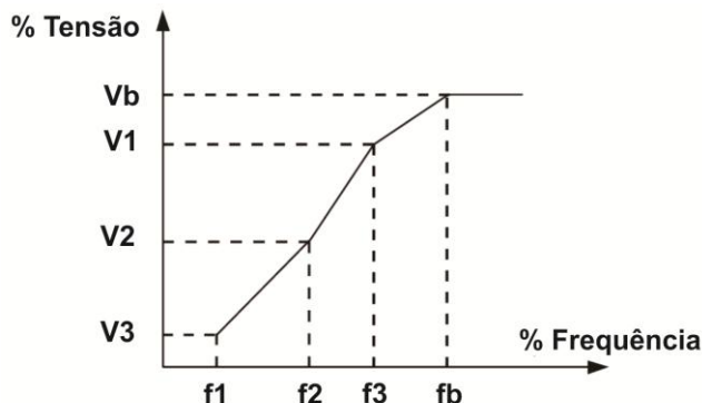
Figura 4-6: Curva multiponto V/F
