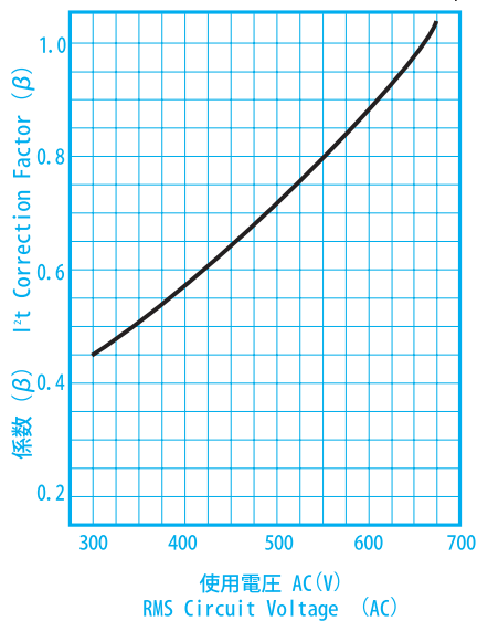
■使用電圧に対する全しゃ断 I^2 t I^2 t Correction Factor (Total I t \times \beta )
